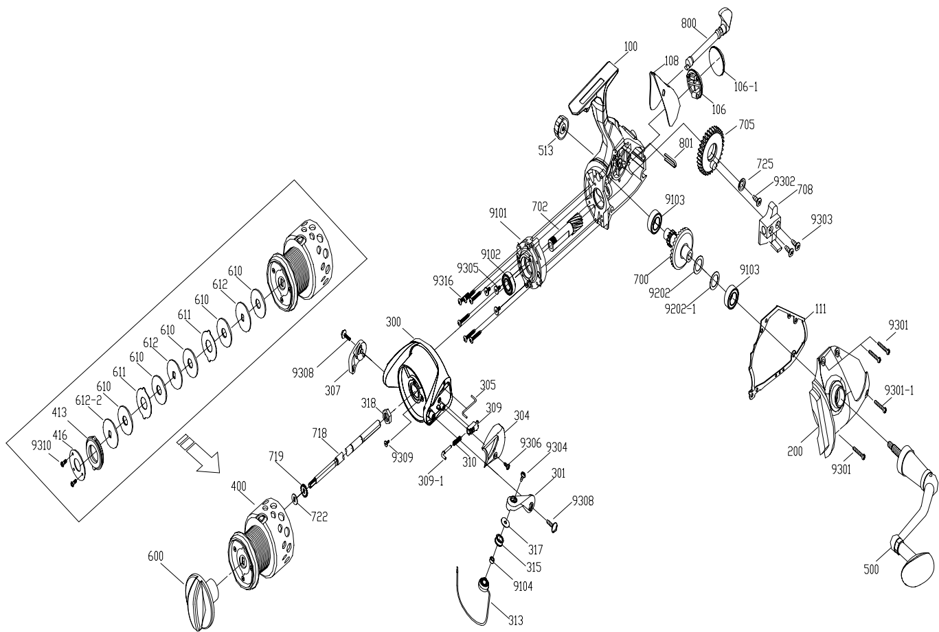
EZ - 65 Spare Parts
